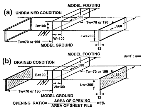
图-2 (a)不透水性矢板、(b)透水性矢板
