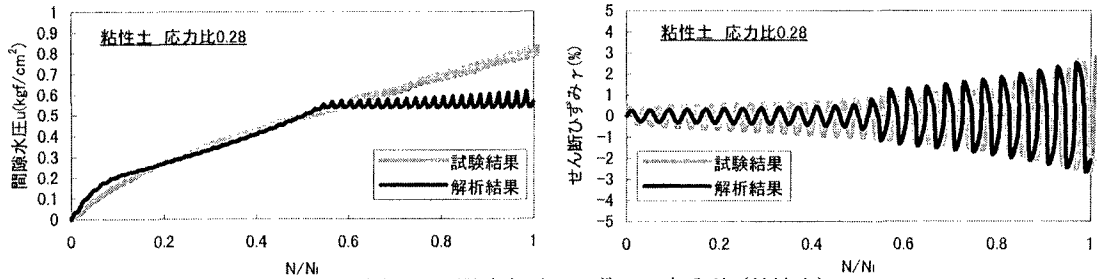
図-5 間隙水圧・ひずみの時系列（粘性土）
