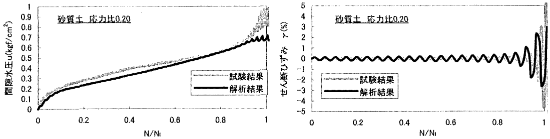
図-3 間隙水圧・ひずみの時系列（砂質土）
