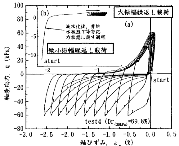
図-5 q と \varepsilon_v の関係(test4)
