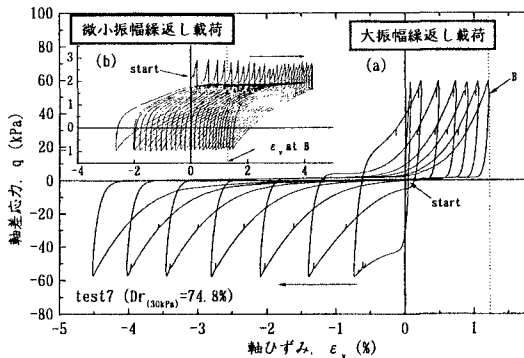
図-2 q と \varepsilon_v の関係(test7)
