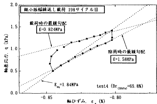
図-6 微小振幅繰返し載荷時のうち最後の198サイクル目の q と \varepsilon_v の関係(test4)
