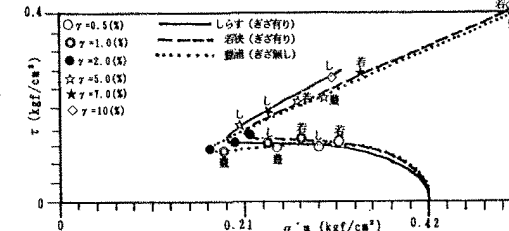
図-6 有効応力経路
