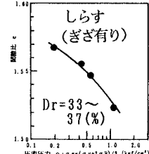
図-2 e \sim \log p 関係
