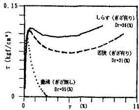
図-3 せん断応力～せん断ひずみ関係
