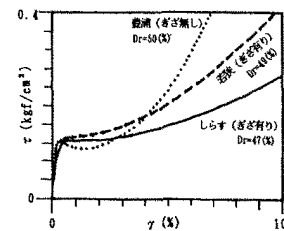
図-5 せん断応力～せん断ひずみ関係
