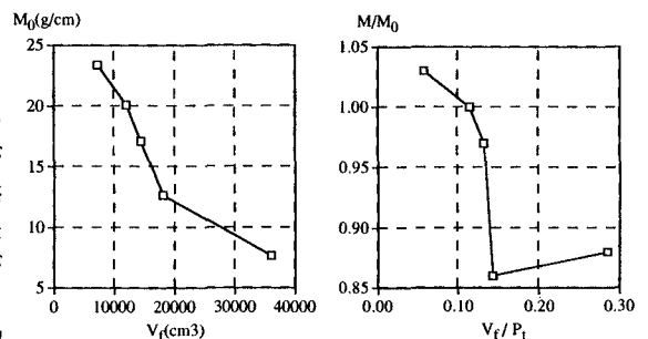
図-4 河川淡水流入体積と塩分侵入量の関係
