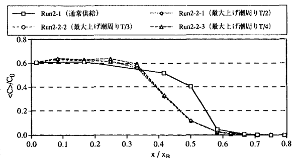
図-3 間断放流を行う時間幅を変えたときの塩水侵入の比較
