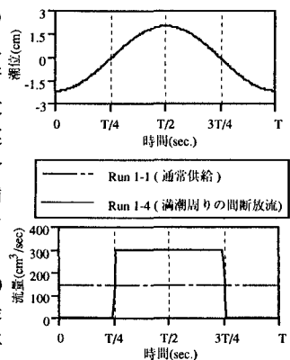
図-1 間断放流時の淡水流量変動パターンの一例(Run1-4)
