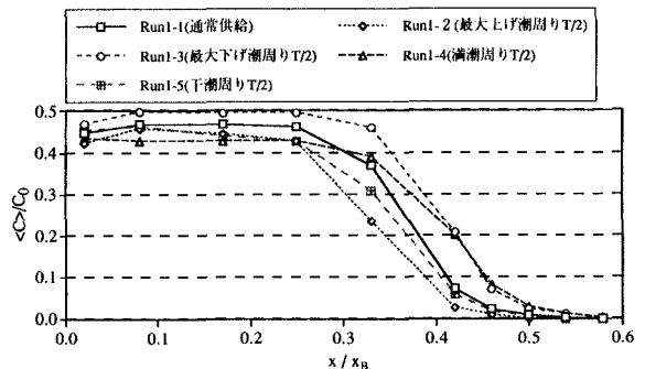
図-2 間断放流の時間幅の違いが塩水侵入に与える影響
