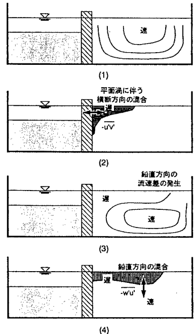
図7 Reynolds 応力 ( -u'w' ) の発生の様式図
