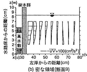
図5 Reynolds 応力分布 ( -u'v' )
