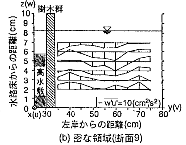
図6 Reynolds 応力分布 ( -w'u' )
