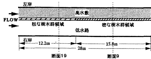
図1 水路平面図
