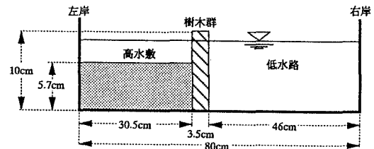
図2 水路横断面図
