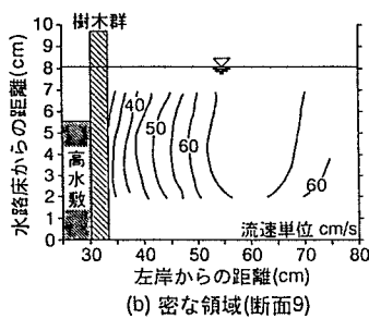
図4 平均流速分布
