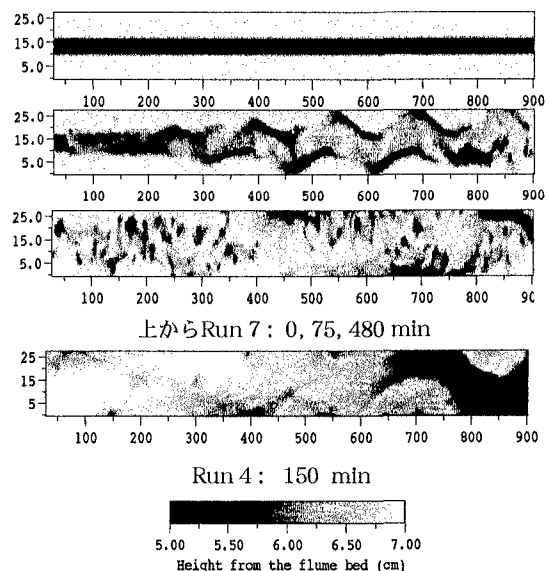
図1 河床形状の変化
