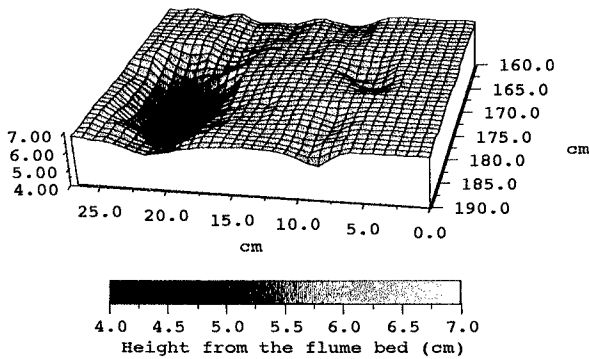
図2 洗掘孔の形状
