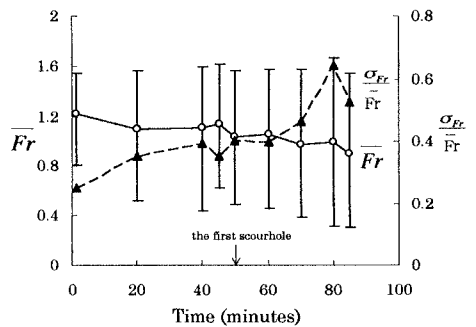
図4 フルード数の平均値と変動係数の変化
