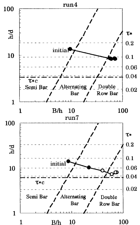
図3 水理量の変化
