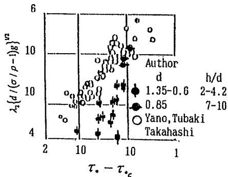
Fig. 1 pickup rate の比較
