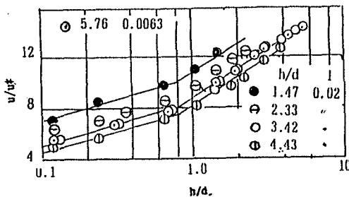
Fig.4 流速分布
