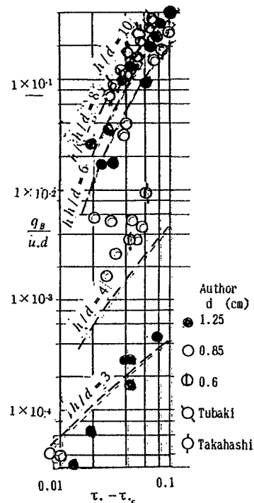
Fig. 3 h/d による流砂量の比較
