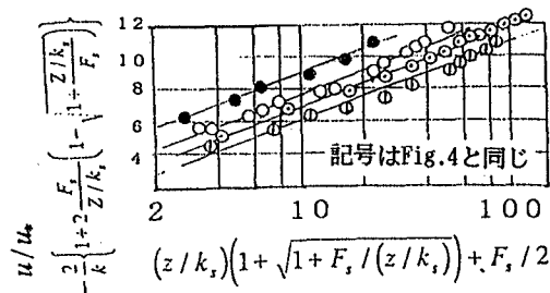
Fig.6 粒子による応力増加を考慮したときの流速分布
