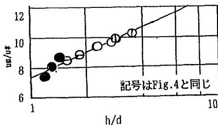
Fig.5 平均流速分布
