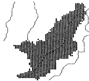
図2: 大戸川上流部流域の抽出
