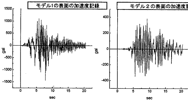
図-3 ポートアイランドの波形を入力した時のモデル表面加速度波形
