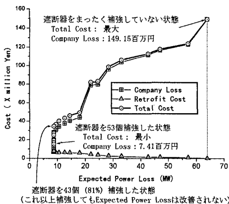
図-4 釧路系統の遮断器 (53 個) を対象とした費用便益分析
