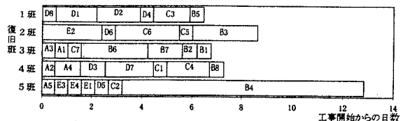
図-4 GAから得られた復旧班の作業日程
