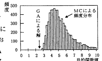
図-5 GAとMCによる目的関数の比較
