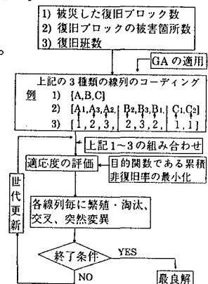
図-1 復旧最適化のための計算フロー
