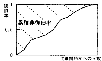
図-2 復旧曲線から求められる累積非復旧率
