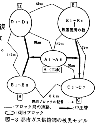
図-3 都市ガス供給網の被災モデル
