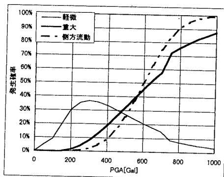
図-3 フラジリティ曲線
