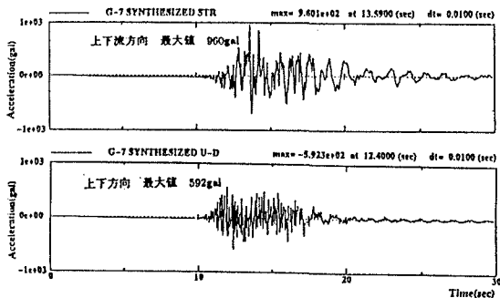
図6 合成した M7.2 地震への応答
