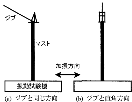
図4 実験概要
