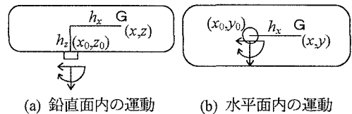
図3 剛体振り子の運動
