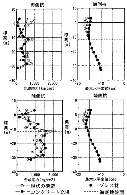
図-4 合成応力と水平変位の深度分布
