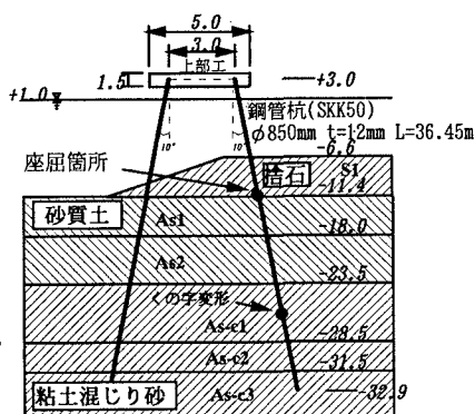
図-1 構造図
