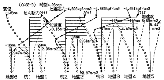
図9 ケースDの解析結果
