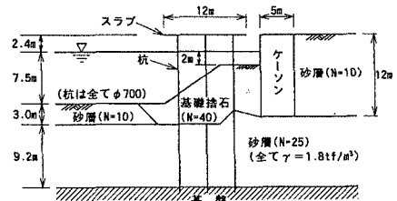
図1 解析対象の横栈橋
