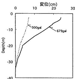
図-4 地盤の最大相対変位
