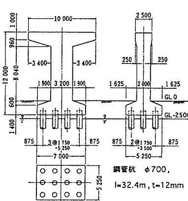
図-1 解析対象橋脚
