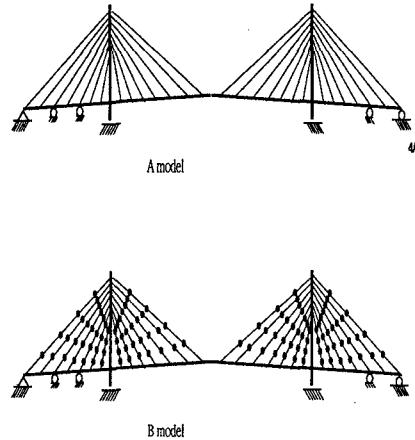
図3 ケーブルのモデル化
