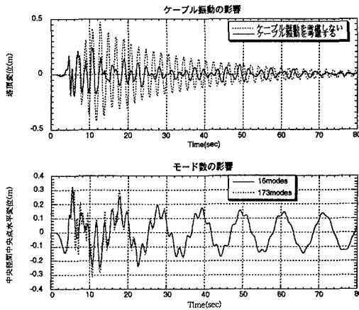
図1 ケーブル振動の影響（上段）
