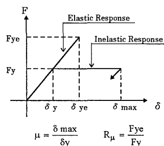
図1 R\mu の計算方法
