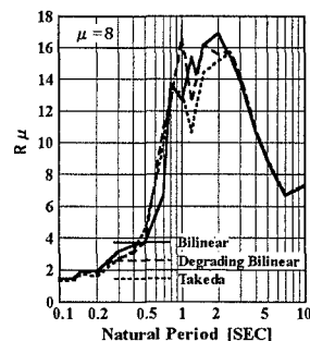
図2 神戸海洋気象台強震記録による各履歴モデルの R\mu スペクトル
