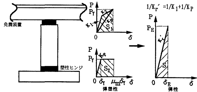
図-1 免震支承をバイリニアモデルとした場合の弾塑性応答
