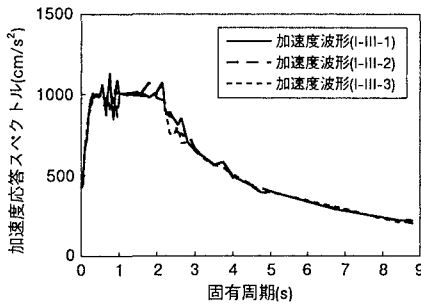
図-2 加速度波形3波の加速度応答スペクトル
