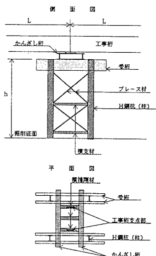
図1 仮橋脚一般図
