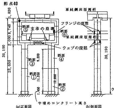
図-1 対象橋脚(寸法単位: mm)
