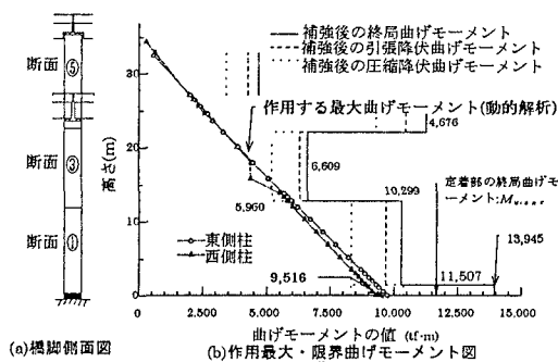
図-4 橋脚断面図と作用・限界曲げモーメント図
