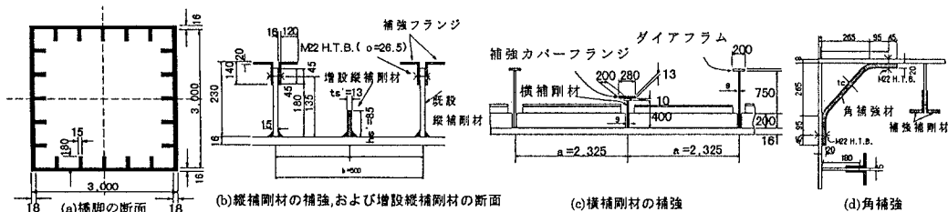
図-3 橋脚柱断面の補強(第③断面) (寸法単位: mm)
