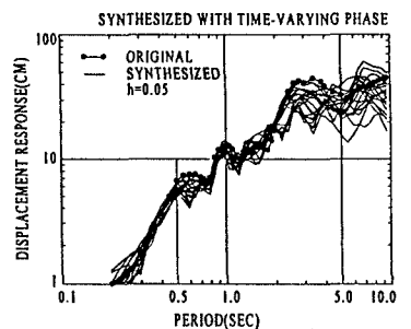
図6 応答スペクトル(バンドパス(1))
