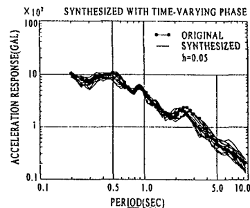
図5 応答スペクトル(バンドパス(3))
