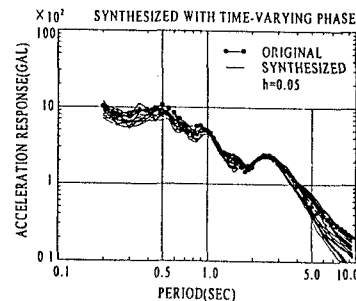
図4 応答スペクトル(バンドパス(2))
