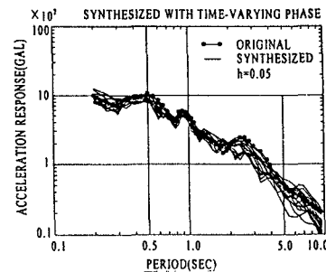
図3 応答スペクトル(バンドパス(1))
