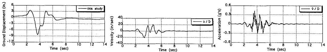
図 5 運動学的断層モデルにと確率論的モデルの合成波形 (左:変位、中央:速度、右:加速度) (0~10 Hz)
