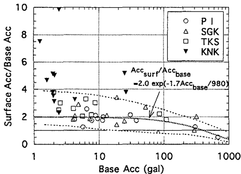
図5 地表と基盤の間での水平加速度増幅率と基盤加速度の関係
