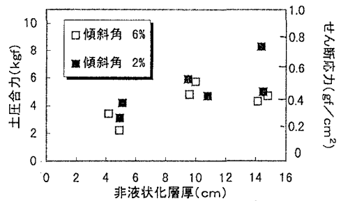
図6. 非液化化層圧と土圧合力およびせん断応力の関係
