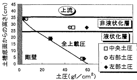
図3. 地中壁に作用する土圧と全上載圧
