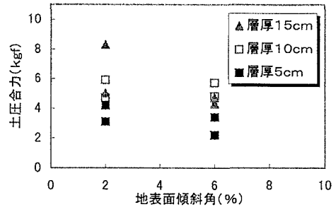
図5. 土圧合力と地表面傾斜角の関係
