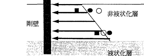
図3. 地中壁に作用する土圧と全上載圧
