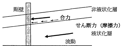
(b) 液化化層と非液化化層の境界面に作用するせん断力
