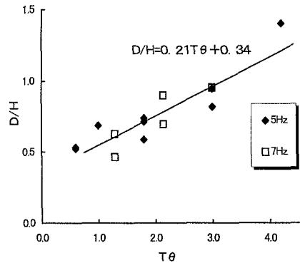
図3 水平変位量÷液状化層厚 ( D/H ) と 入力波の継続時間×傾斜角 ( T\theta ) の関係
