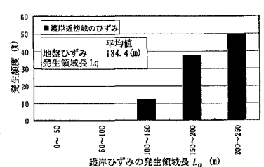
図9 護岸近傍域における地盤ひずみの発生領域長
