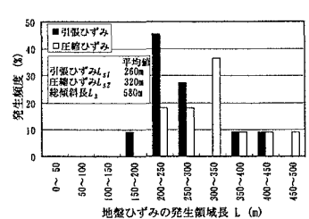
図6 傾斜地盤における地盤ひずみの発生領域長
