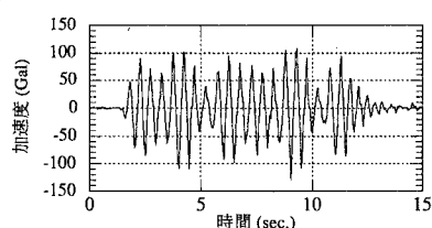
図2 入力加速度時刻歴（ A_{\max}=130\text{Gal} ）
