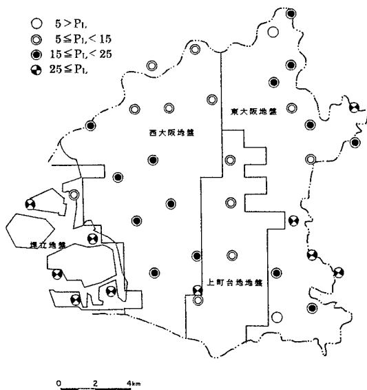
図-3 各地点の P_L 値
