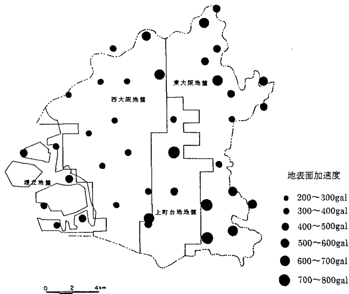
図-1 地震動の算定地点と加速度分布
