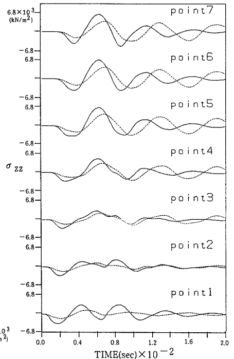
図4 鉛直応力の時刻歴応答 ( V_0 = 100 cine)
