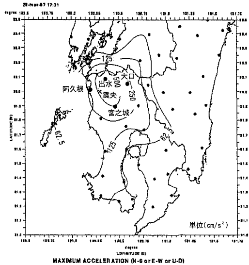
図-1 K-NetによるPGA分布と震央の四方に位置する観測地点(K-Netの最大加速度分布図に加算)
