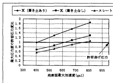
図4 地表面加速度と最大応力の関係
