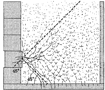
図-6 接触力分布(衝突速度1m/s)
