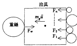
図-5 移動治具の力のつり合い
