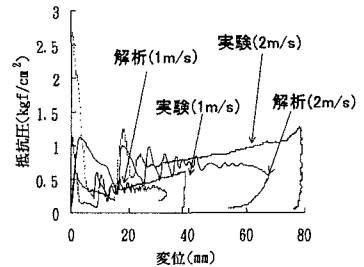
図-7 緩詰め抵抗圧～変位関係
