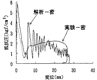
図-8 密詰め抵抗圧～変位関係 (衝突速度2m/s)
