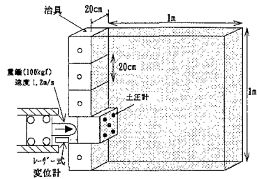
図-1 衝撃実験装置
