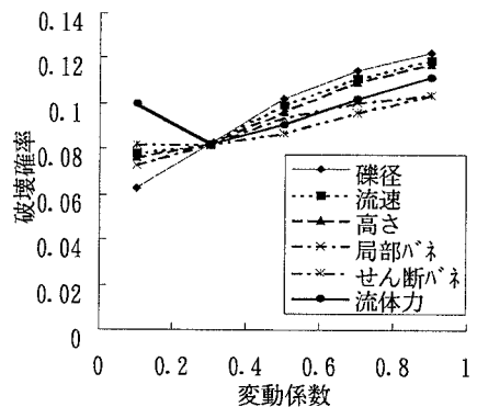
図—4 変動係数と破壊確率の関係
