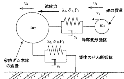
図-1 2質点バネモデル
