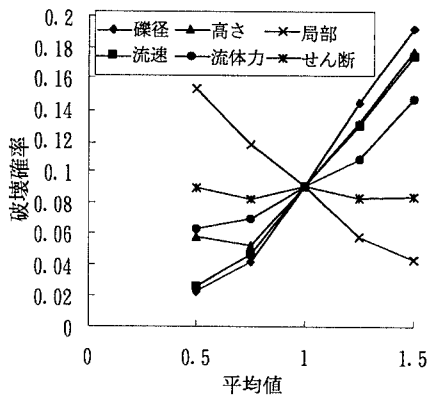
図—5 平均値と破壊確率の関係
