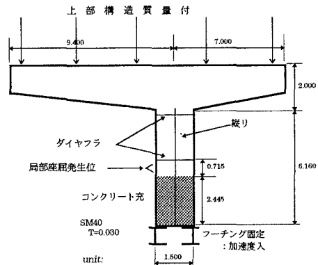
図2 矩形断面橋脚（P-353）
