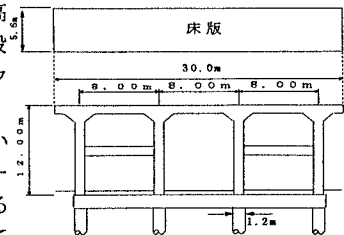
図-1 一般図
