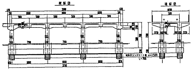
図-2 一般図
