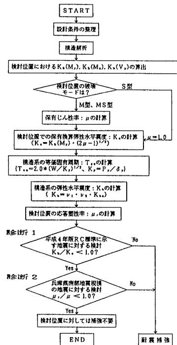
図-1 耐震診断フローチャート
