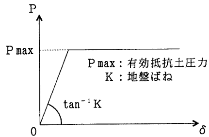
図3 地盤ばねの非線形モデル
