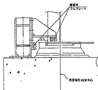
図-1 鋳鉄沓標準補強図
