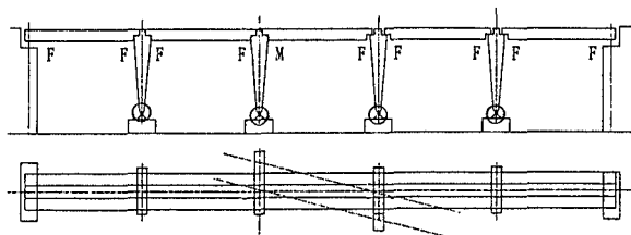
図-2 受け梁を有する跨線橋
