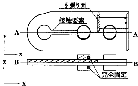
図3 解析モデル
