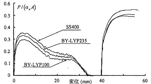
図 5-(a) スリット幅が 6mm の形状の比較
