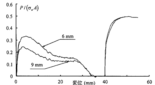
図 5-(d) BY-LYP235 でスリット幅の異なるものの比較
