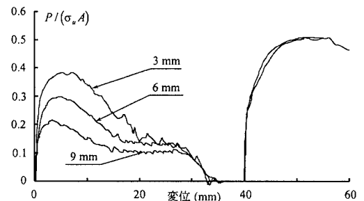
図 5-(c) BY-LYP100 でスリット幅の異なるものの比較
