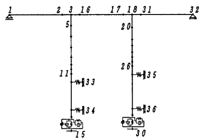
図4(a) 解析モデル1(剛結)
