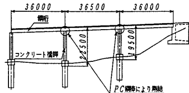
図1 一般図
