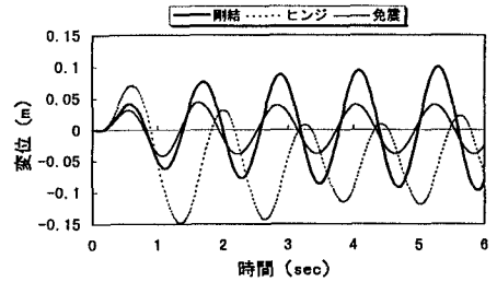
図5 時刻歴応答変位(節点3)
