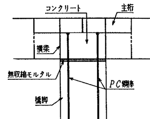
図2 剛結部
