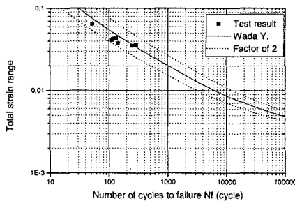
図 4：S-N 曲線
