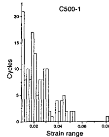
図 5：ひずみ範囲のヒストグラム
