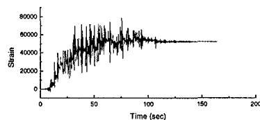
図3：ひずみ履歴(解析結果)
