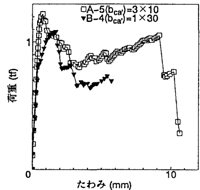
図4 荷重-たわみ曲線( b_{ca}=30 )
