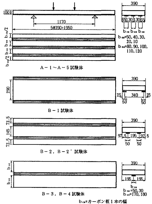
図1 試験体 (単位: mm)
