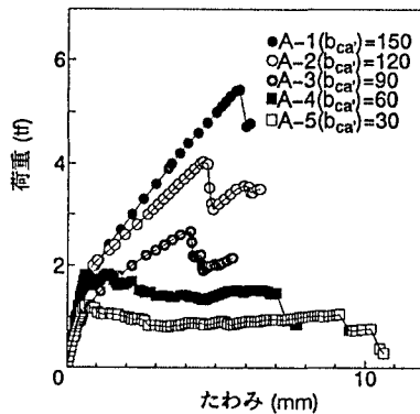
図2 Aシリーズの荷重-たわみ曲線
