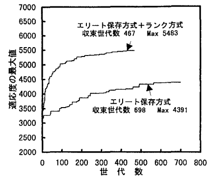
図-2 選択処理の違いによる適応度の収束性及び最適解の比較
