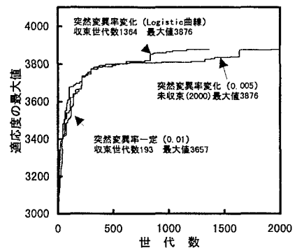
図-3 突然変異処理の違いによる適応度の収束性及び最適解の比較
