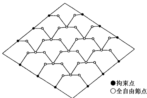
図-1 初期形状(鳥瞰図)
