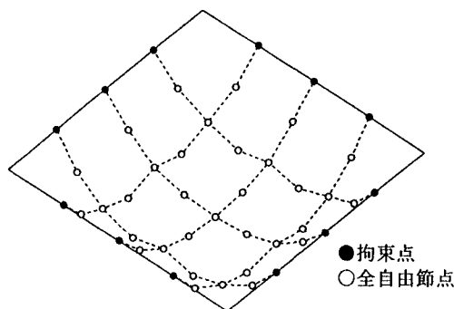
図-2 最終形状(鳥瞰図)
