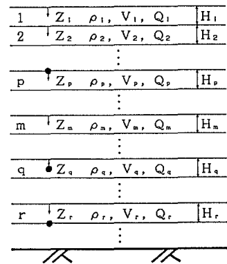
図-1 地盤モデル
