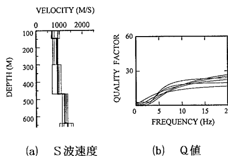
図-3 同定結果（富岡観測点）
