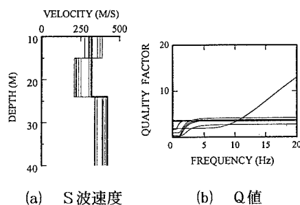
図-2 同定結果 (東京大学生産技術研究所)
