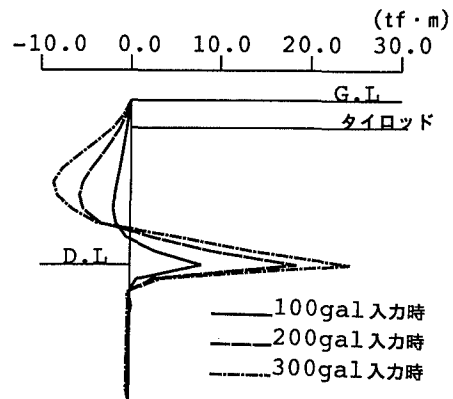
図-2 最大応答曲げモーメント
